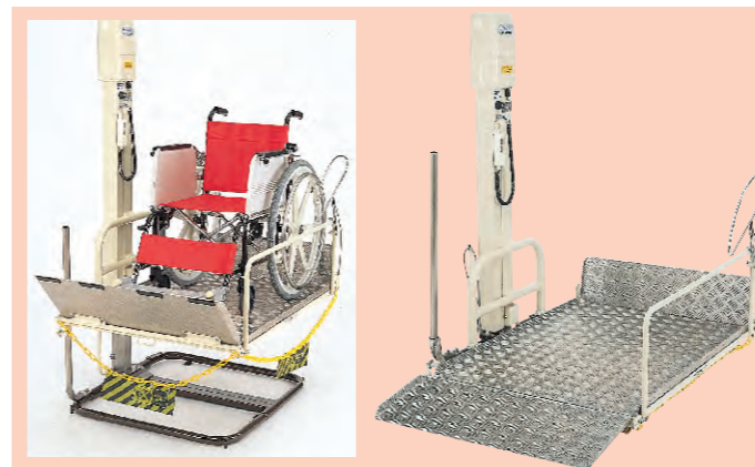
全高 76~118cm 幅53cm 奥行60.5cm
